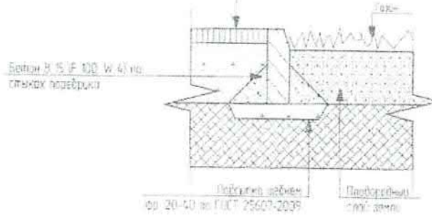
Узел конструкции пешеходной дорожки Тип 3
